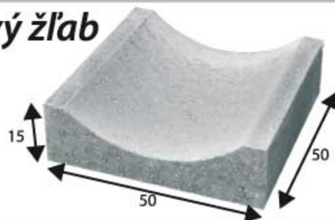
Betónový žľab
