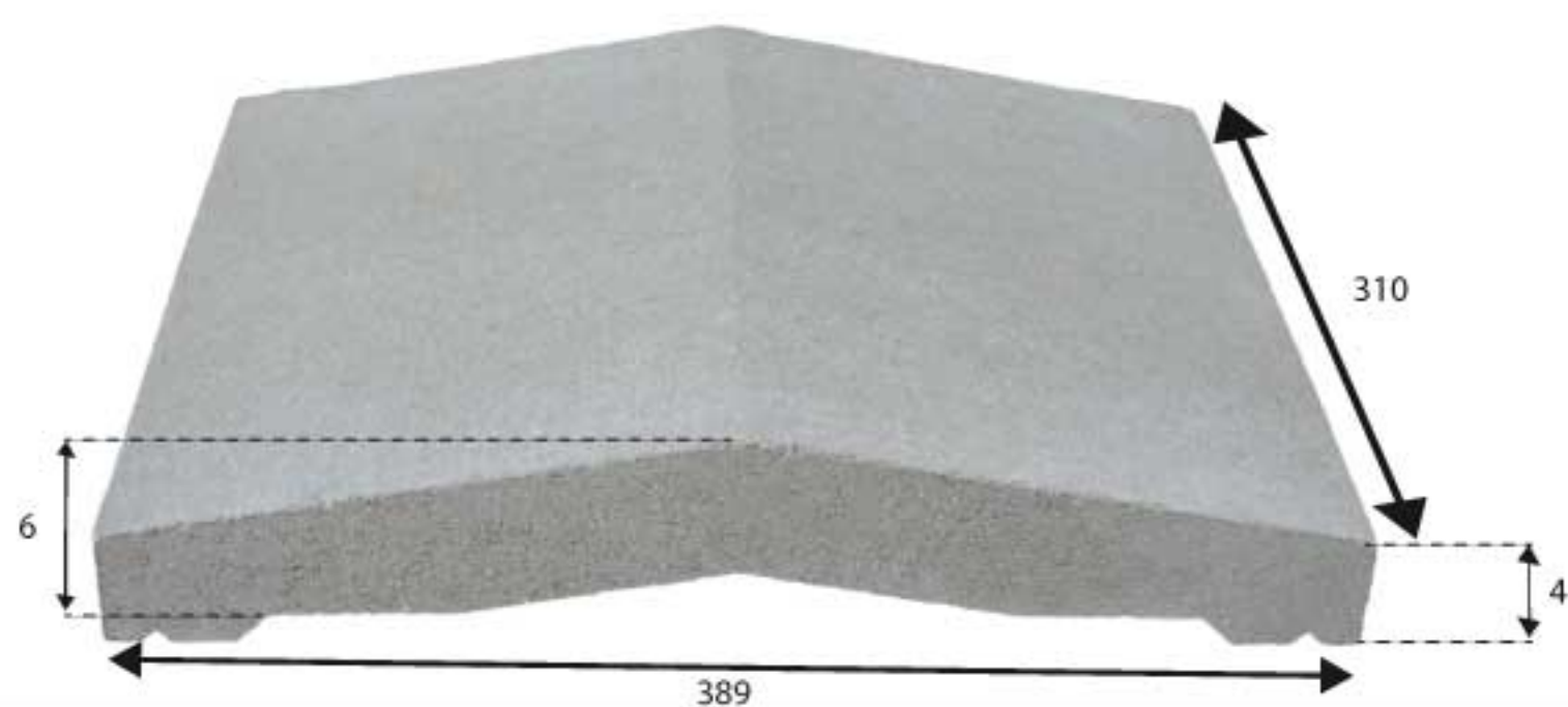
Strieška múriková
