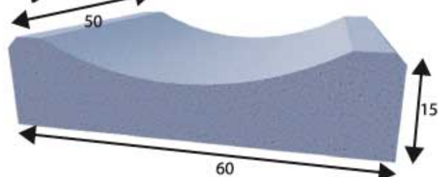
Betónový žľab
